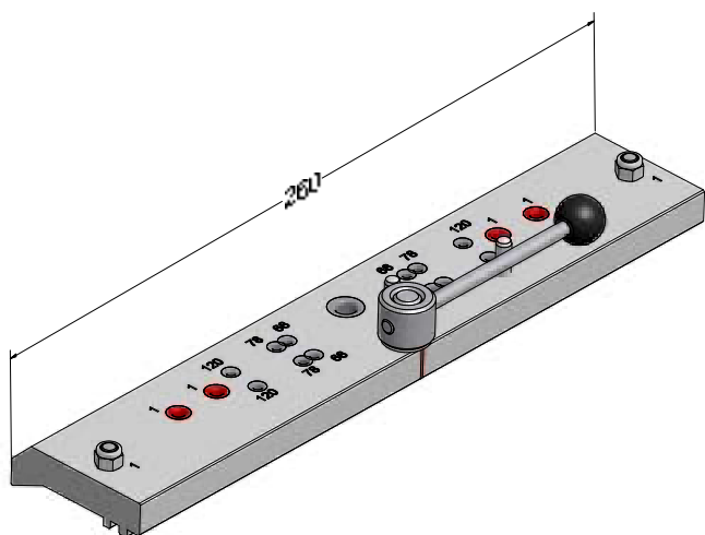
Шаблон (для установки горбылька 68, импоста 78 в створку)
