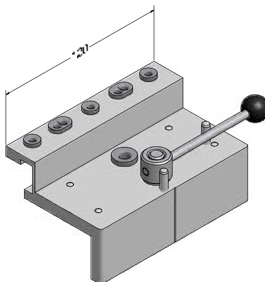
Шаблон (для установки фиксаторов горбылька 68 в створку)
